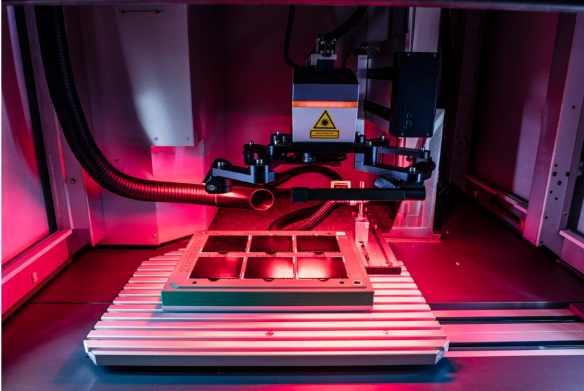
Bestandteil der vollautomatisierten Fertigungslinie für Busch-tacteo® ist die Laserbearbeitung: Der Träger fasst bis zu sechs Bedienelemente zusammen.
