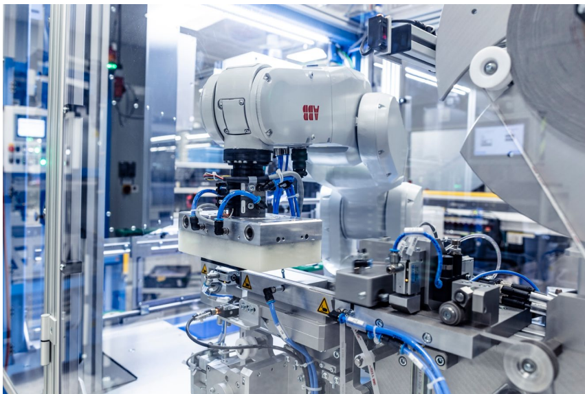
Für die Verklebung von Glaspaneel und Gehäuse sind moderne Industrie-Roboter zuständig.
