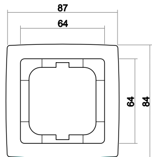
Abdeckrahmen 1-fach
