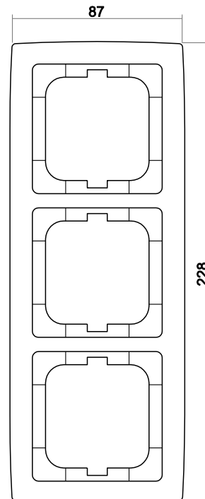
Abdeckrahmen 3-fach
