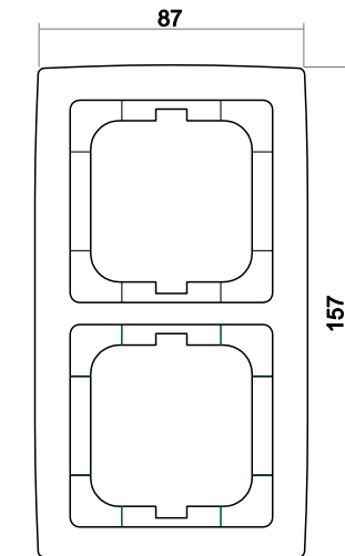
Abdeckrahmen 2-fach
