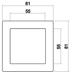
Schalter 1-fach
