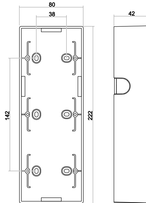
AP-Gehäuse 3-fach
