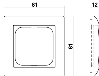
Abdeckrahmen 1-fach
