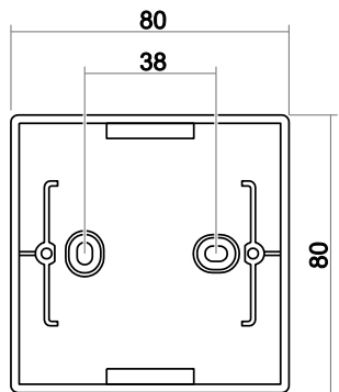
AP-Gehäuse 1-fach
