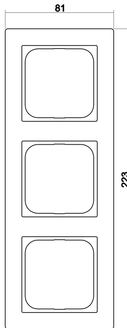
Abdeckrahmen 3-fach
