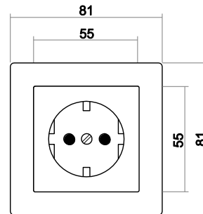
Steckdose 1-fach
