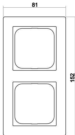
Abdeckrahmen 2-fach
