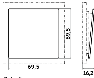
Schalter
