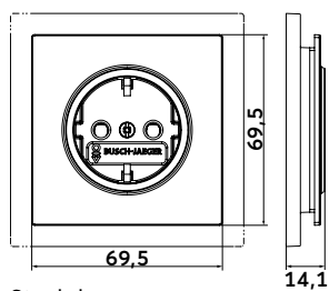
Steckdose
