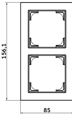
Abdeckrahmen 2-fach
