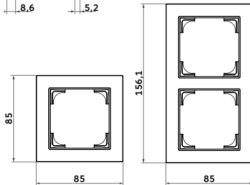
Abdeckrahmen 1-fach
