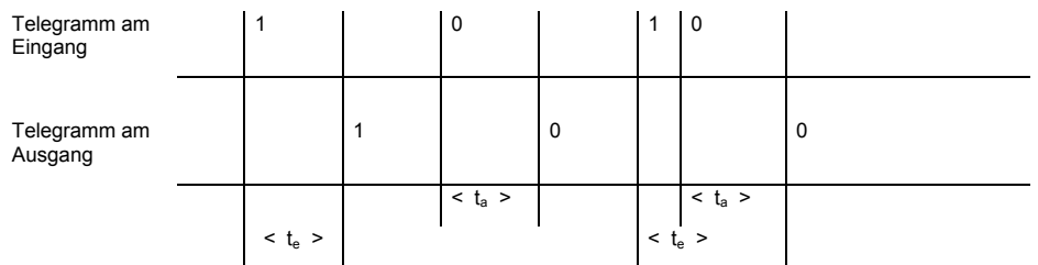
Abb. 80: Diagramm „Ein- und Ausschaltverzögerung“
