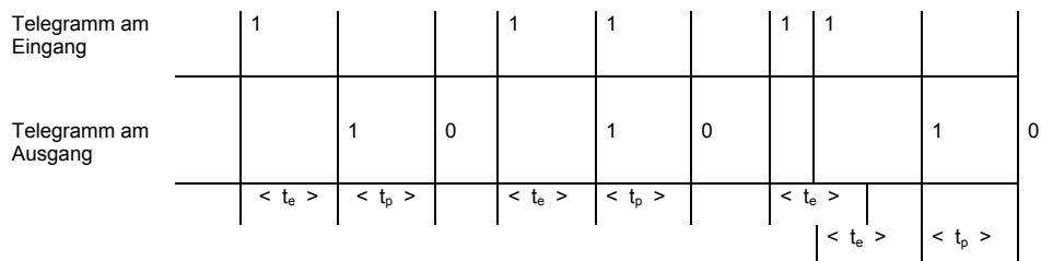
Abb. 84: Diagramm "Einschaltverzögerung und Impulsdauer"
