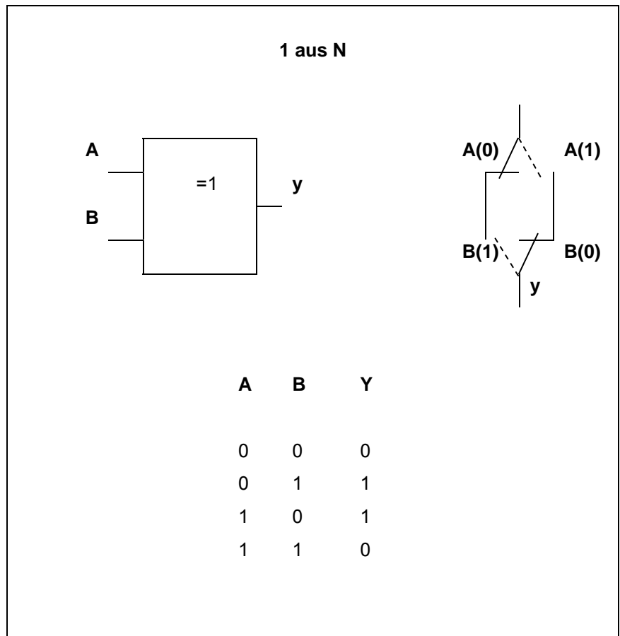
Abb. 66: 1 aus N – Wahrheitstabelle 2 Eingänge
