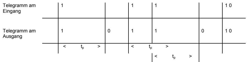
Abb. 82: Diagramm "Impulsdauer"
