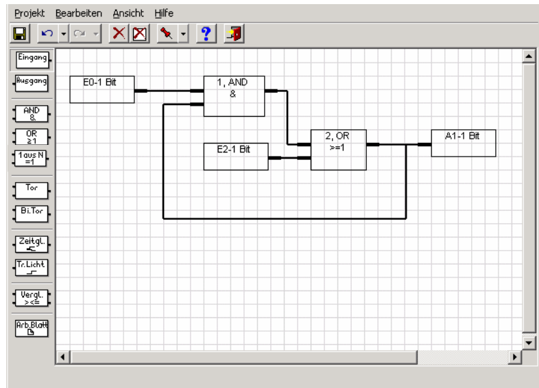
Abb. 56: Beispiel Rückkopplung
