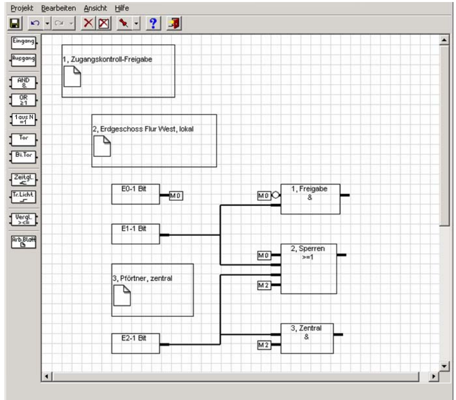
Abb. 93: Anzeige von Arbeitsblättern
