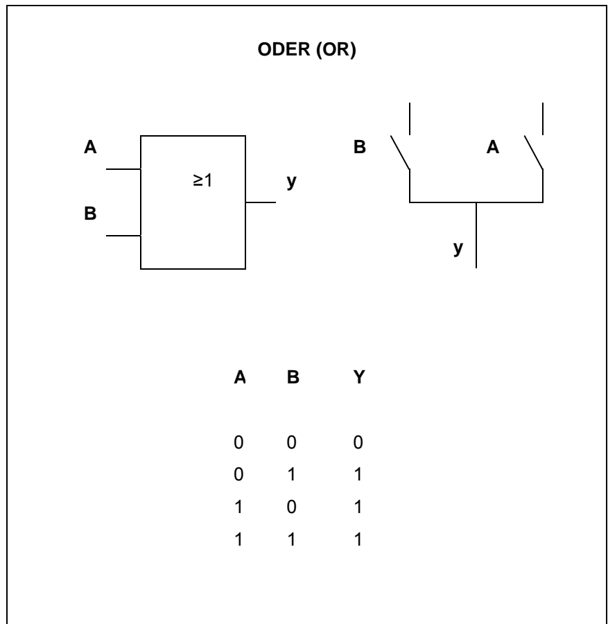
Abb. 63: ODER (OR) - Wahrheitstabelle
