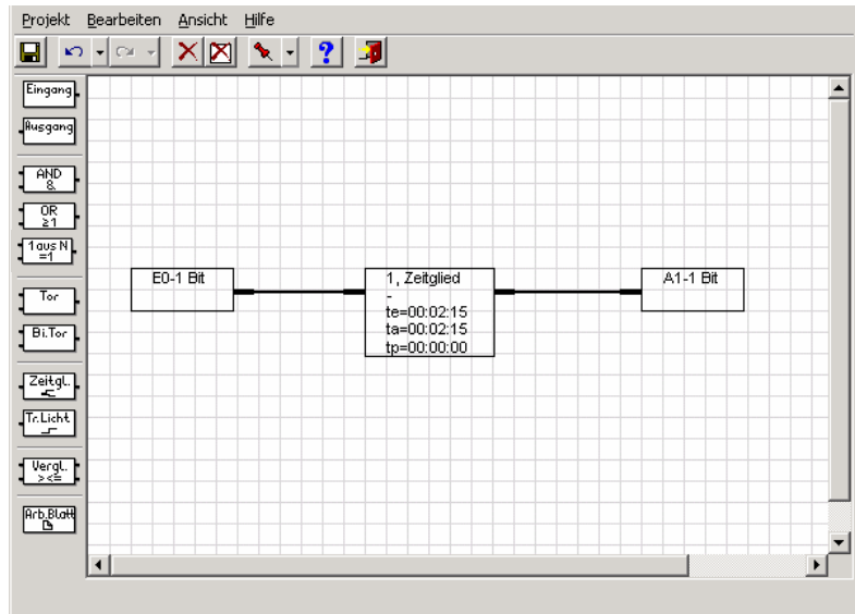
Abb. 79: Ein- und Ausschaltverzögerung
