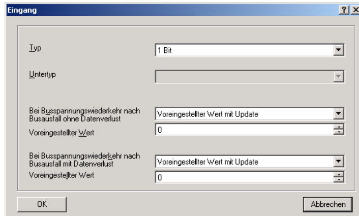
Abb. 51: Parameterfenster „Eingang“
