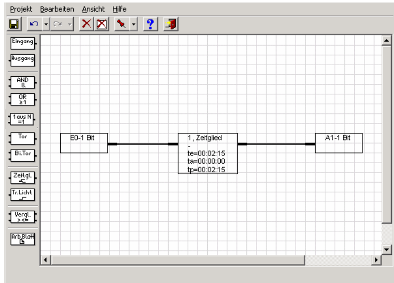
Abb. 83: Einschaltverzögerung und Impulsdauer
