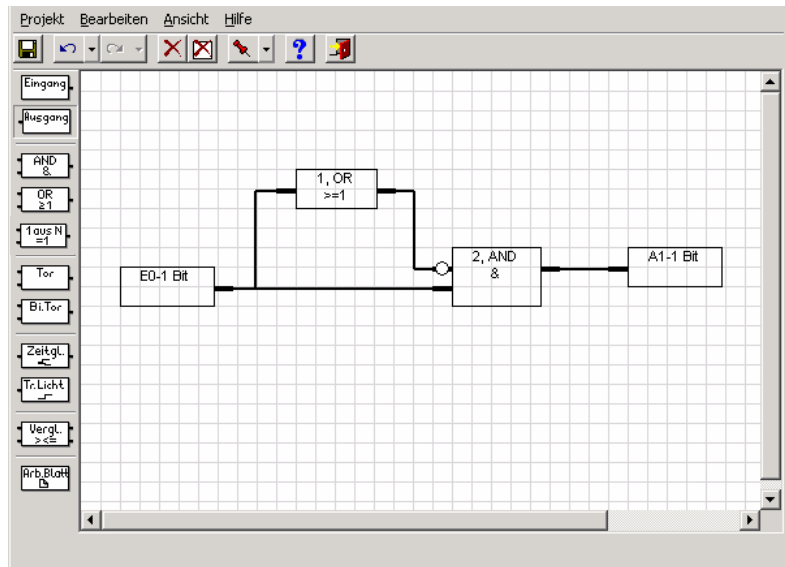
Abb. 99: Keine Glitches
