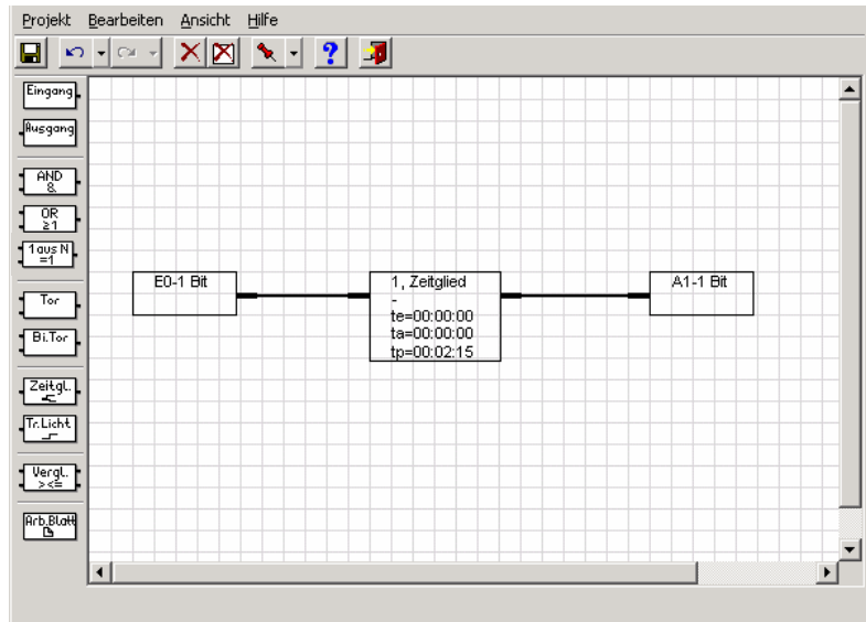
Abb. 81: Impulsdauer
