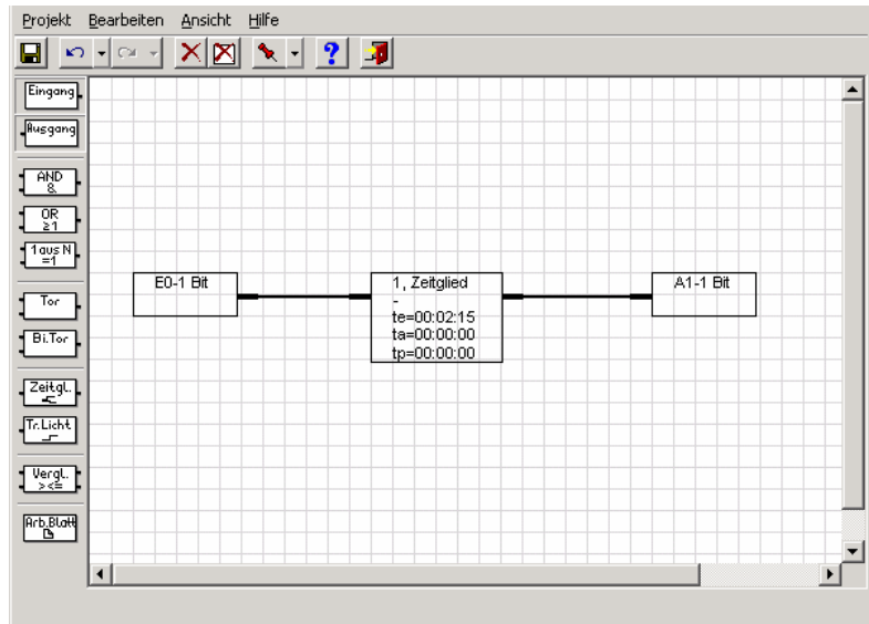
Abb. 75: Einschaltverzögerung
