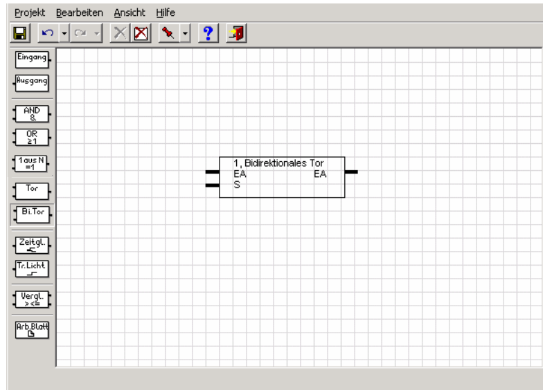
Abb. 71: Bidirektionales Tor
