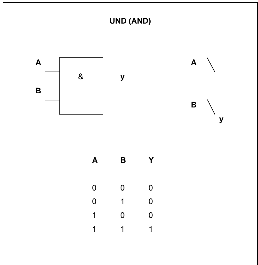
Abb. 60: UND(AND) - Wahrheitstabelle
