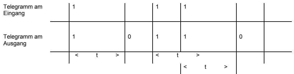
Abb. 87: Diagramm "Treppenlicht-Funktion"
