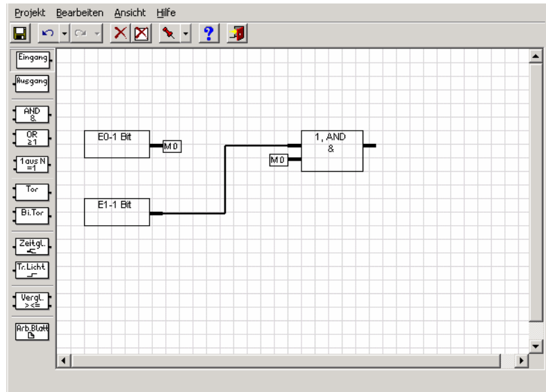
Abb. 47: Verbinden von Funktionen
