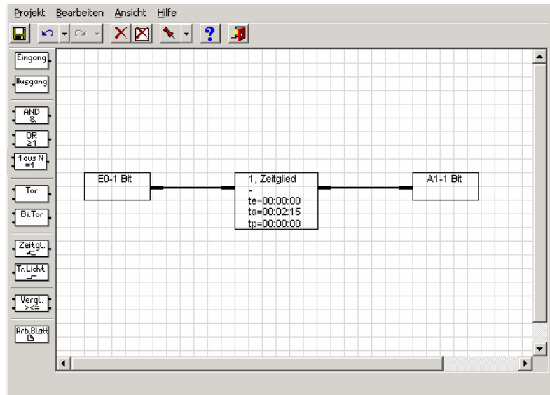
Abb. 77: Ausschaltverzögerung
