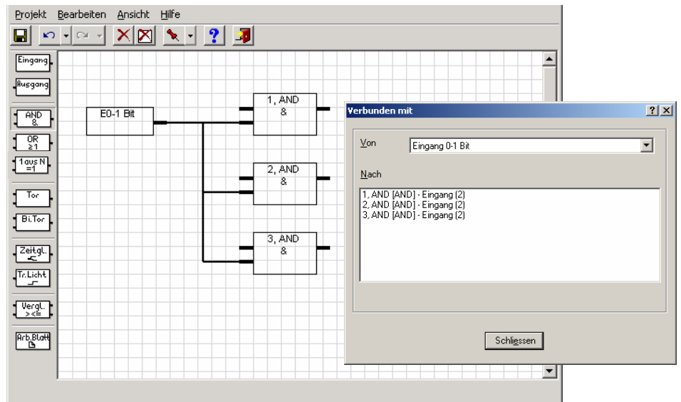
Abb. 49: Anzeigen von Verbindungen
