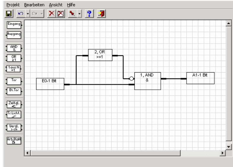
Abb. 98: Glitches
