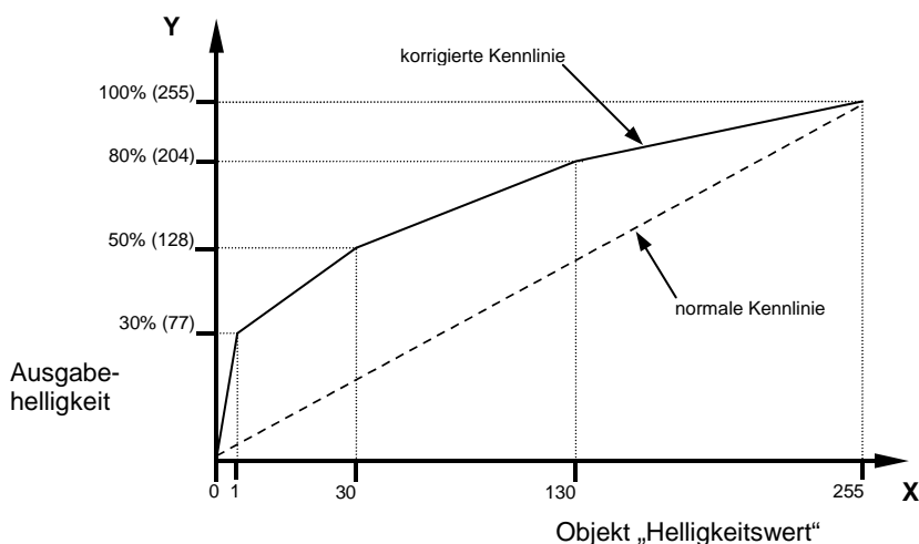
Abbildung 1: Beispiel für eine Kennlinienkorrektur
