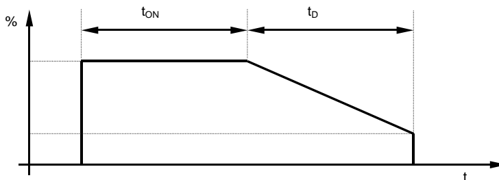
Abbildung 2: Zeitverlauf der Helligkeit bei Treppenlicht
