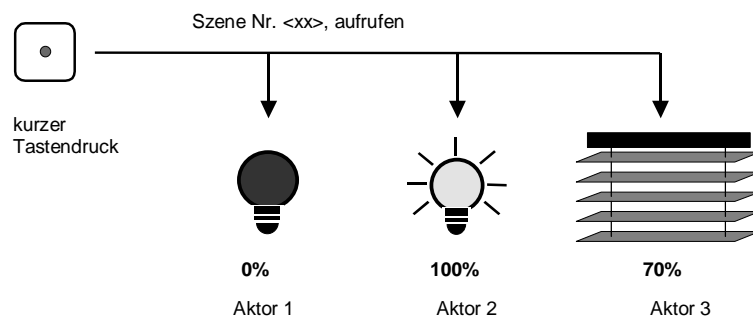
Abb. 1 : Szene aufrufen, 8-Bit-Szene
