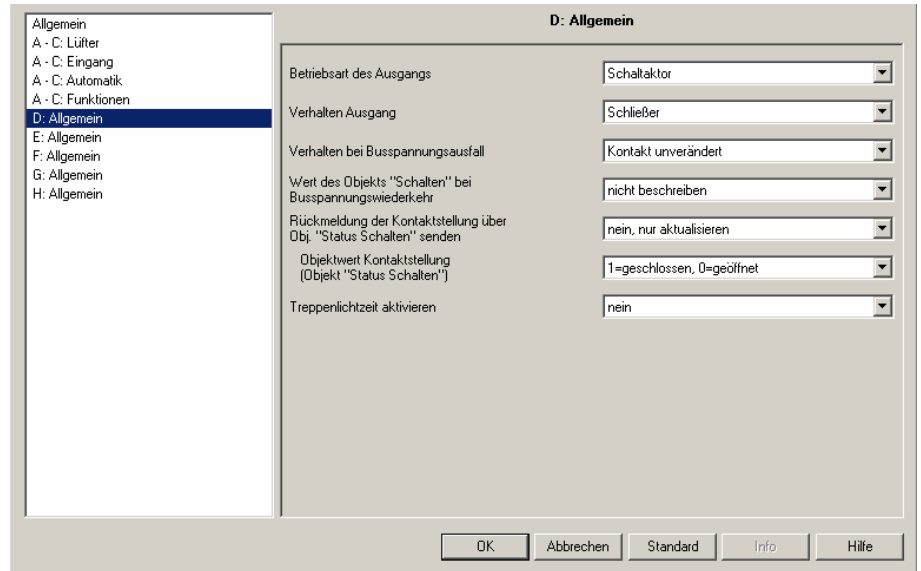
Abb. 20: Parameterfenster "D: Allgemein" - Schaltaktor
