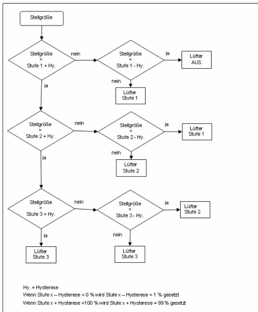
Abb. 35: Logik Lüfterstufenumschaltung
