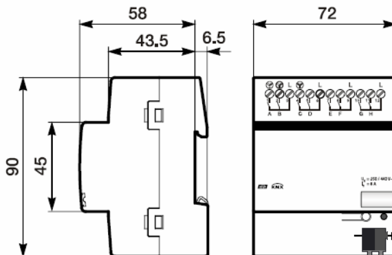
Abb. 7: Maßbild 6164/42
