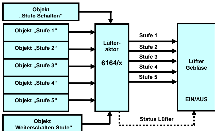
Abb. 25 Prinzipschaltbild Lüfteransteuerung über EIB / KNX
