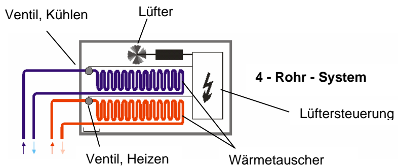
Abb. 32: Aufbau 4-Rohr Fan Coil - Einheit
