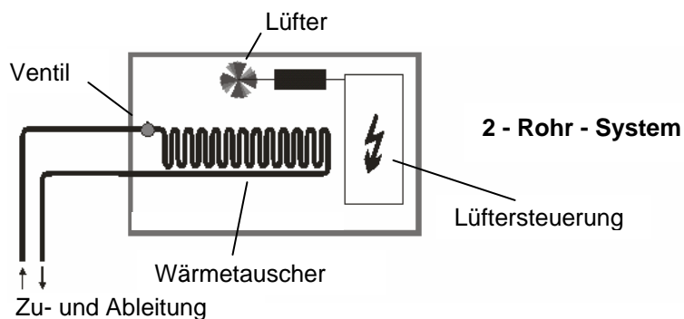
Abb. 27: Aufbau 2-Rohr Fan Coil – Einheit (Unit)
