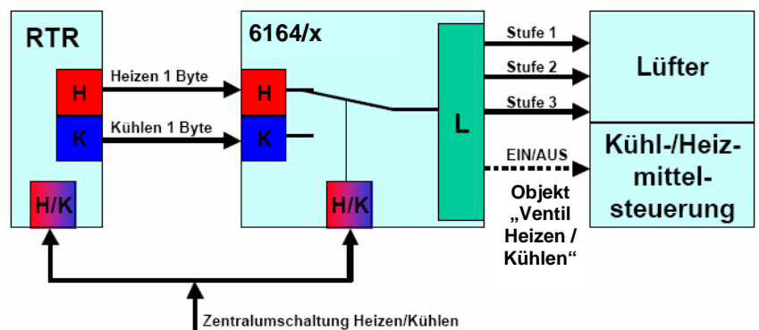
Abb. 28: Prinzipschaltbild 2-Rohr-System Heizen und Kühlen (3stufiger Lüfter)
