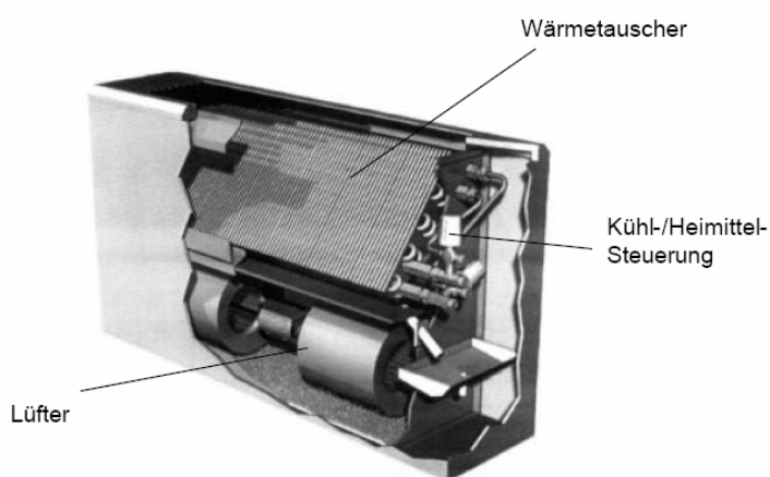
Abb. 26: Beispiel Gebläsekonvektor
