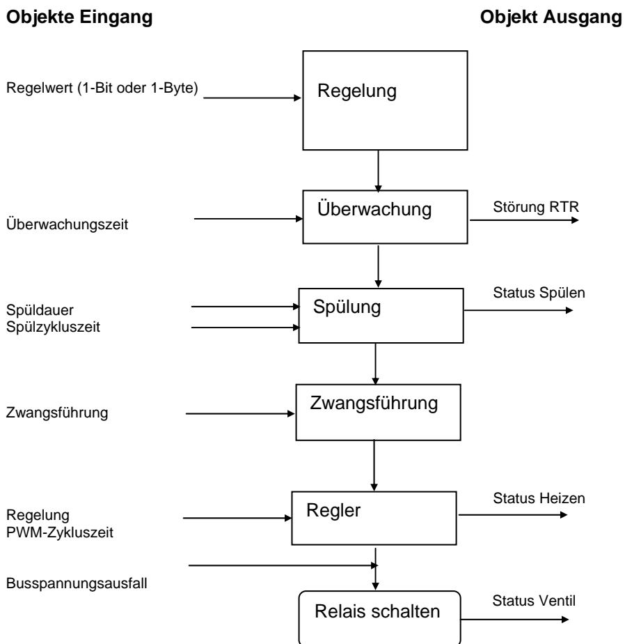
Abb. 38: Funktionsschaltbild – Steuerung Ventil (Heizung)
