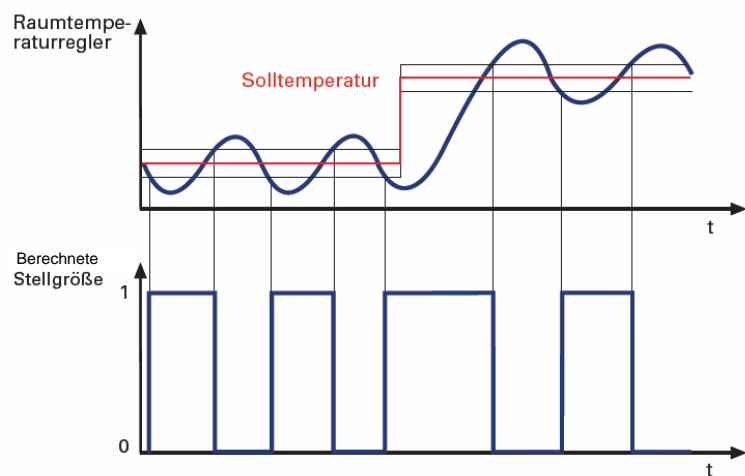
Abb. 39: Diagramm 2-Punkt Regelung
