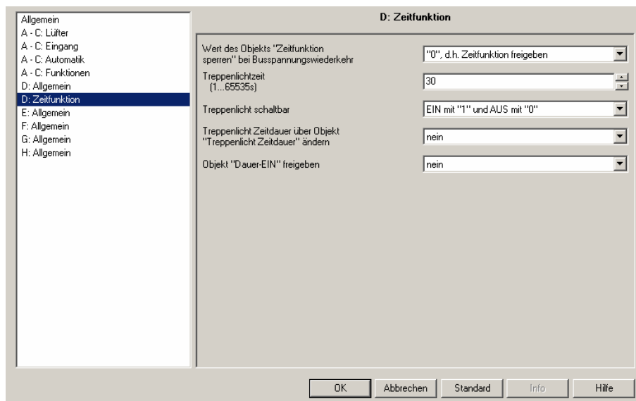
Abb. 21: Parameterfenster "D: Zeitfunktion" - Schaltaktor
