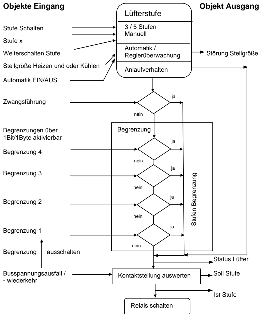
Abb. 36: Funktionsschaltbild Begrenzungen des Schaltaktors
