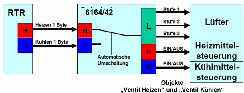
Abb. 33: Prinzipschaltbild 4-Rohr-System (3stufiger Lüfter)
