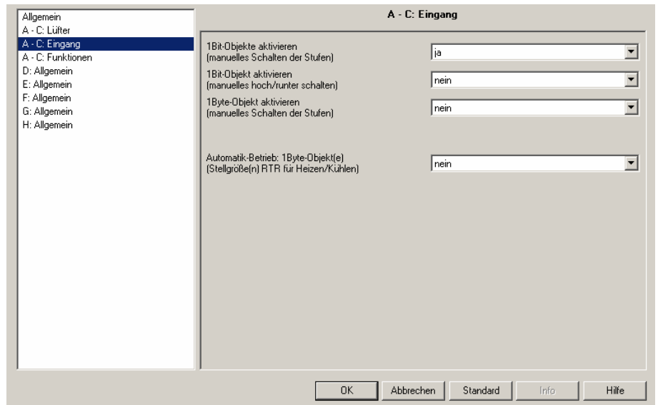
Abb. 11: Parameterfenster " A - C: Eingang"
