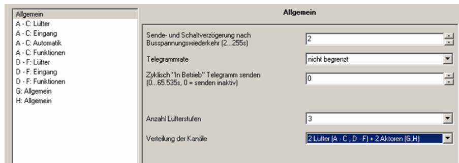
Abb. 17: Parameterfenster "Allgemein", zwei Lüfter
