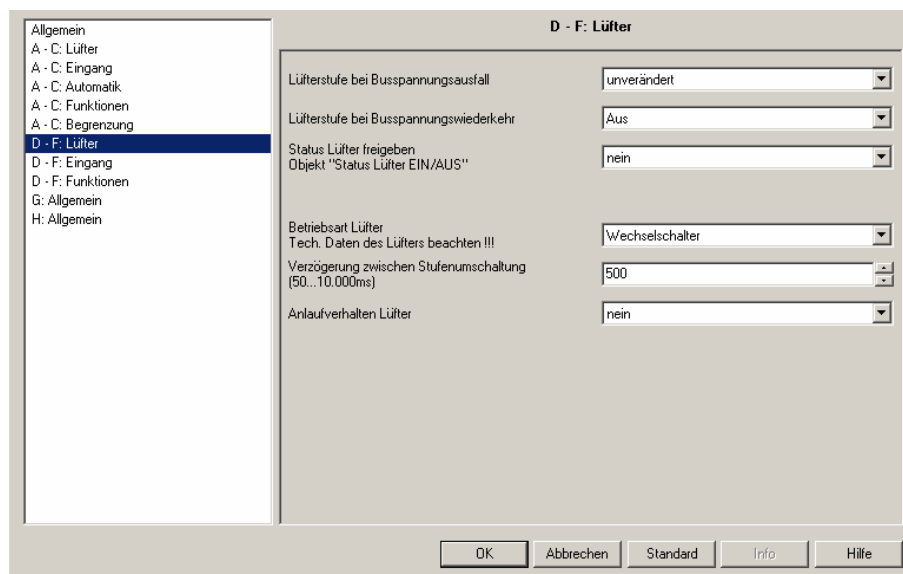
Abb. 16: Parameterfenster "D - F: Lüfter"
