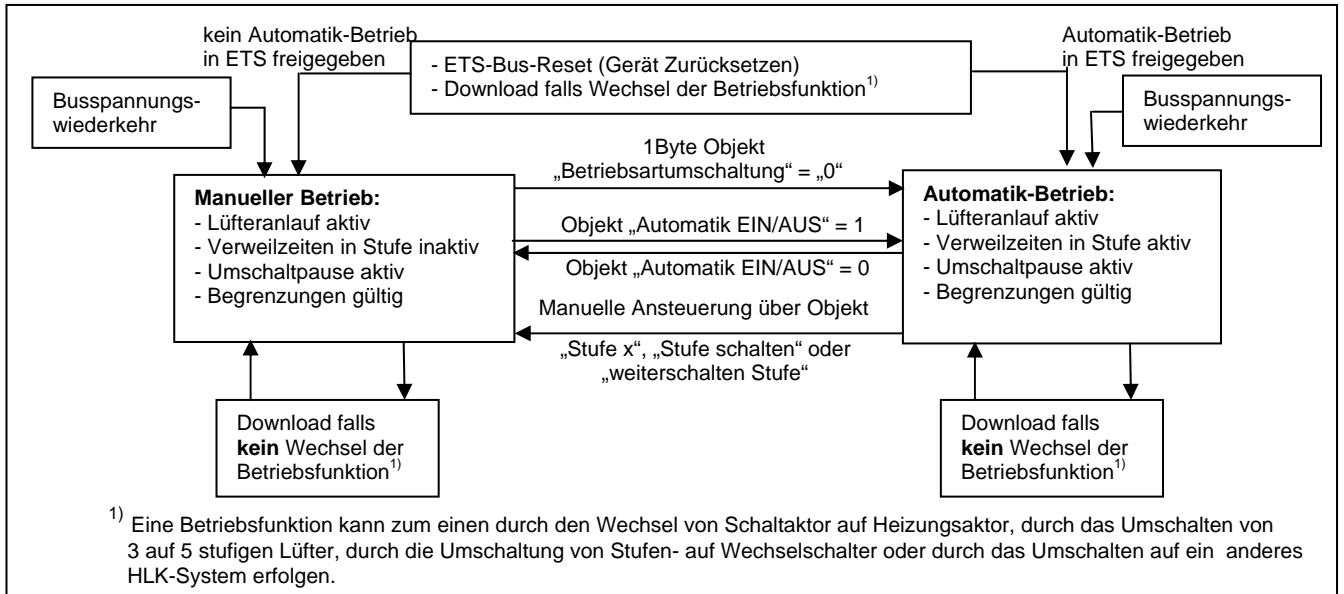
Abb. 34: Funktionsschaltbild Automatik-Betrieb
