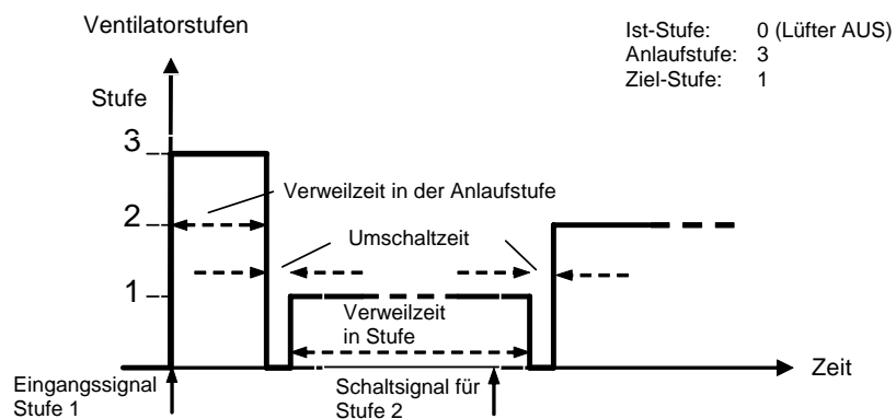
Abb. 10: Anlaufverhalten eines Lüfters
