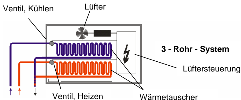
Abb. 31: Aufbau 3-Rohr Fan Coil - Einheit
