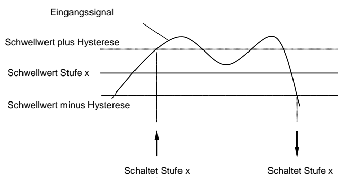
Abb. 13: Hysterese bei Lüftersteuerung
