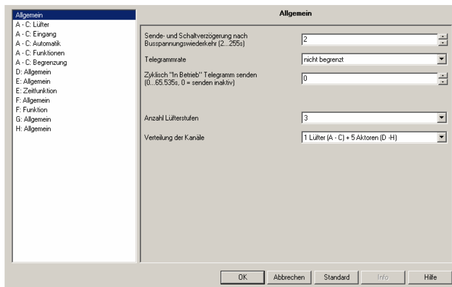
Abb. 8: Parameterfenster „Allgemein“
