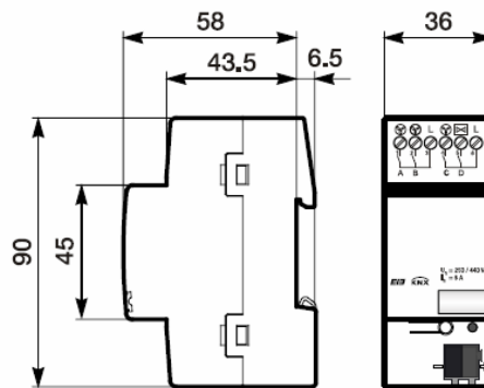
Abb. 4: Maßbild 6164/41
