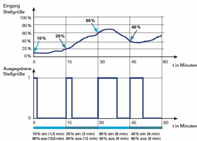
Abb. 40: Diagramm PWM Regelung
