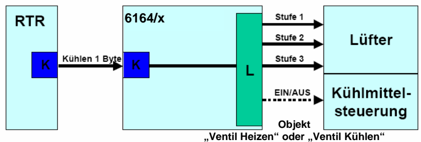
Abb. 29: Prinzipschaltbild 2-Rohr-System Heizen oder Kühlen (Abgebildet Kühlen, 3stufig)
