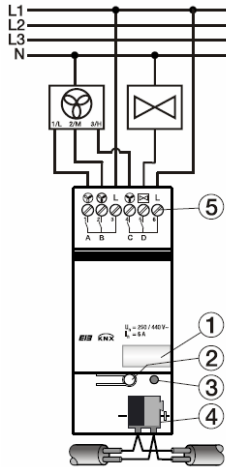
Abb. 3: Anschlussbild des Lüftungsaktors, 3stufig 6164/41
