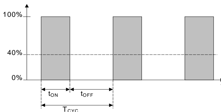
Abb. 41: Diagramm PWM Berechnung
