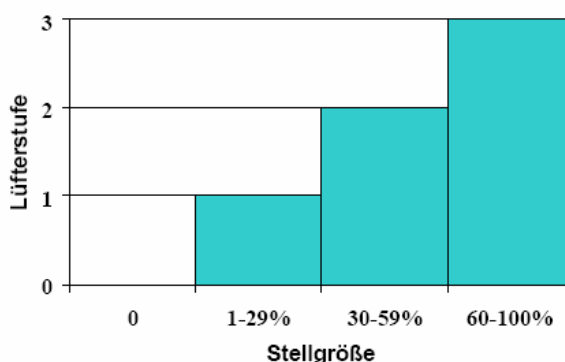
Abb. 30: Funktionsdiagramm Fan Coil 2-Rohr-System (3stufiger Lüfter)
