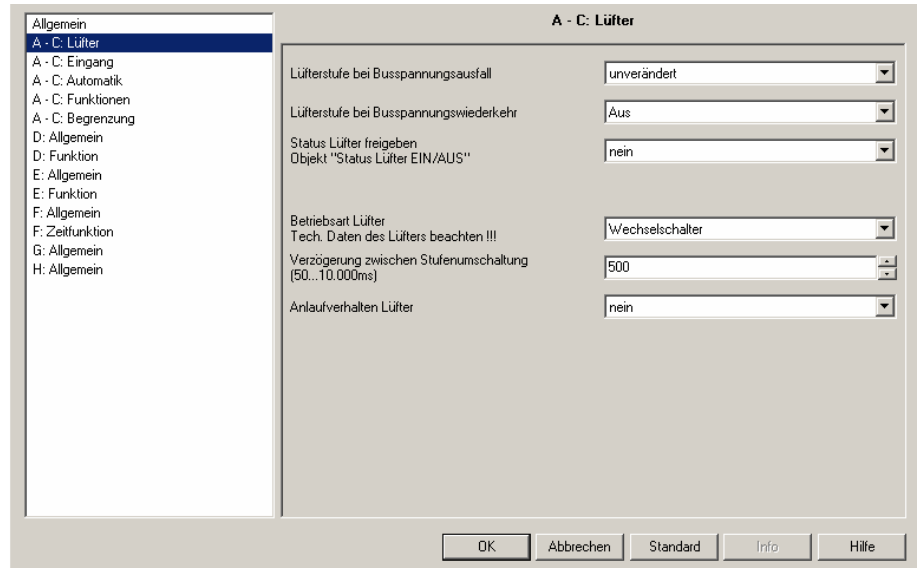
Abb. 9: Parameterfenster " A - C: Lüfter"
