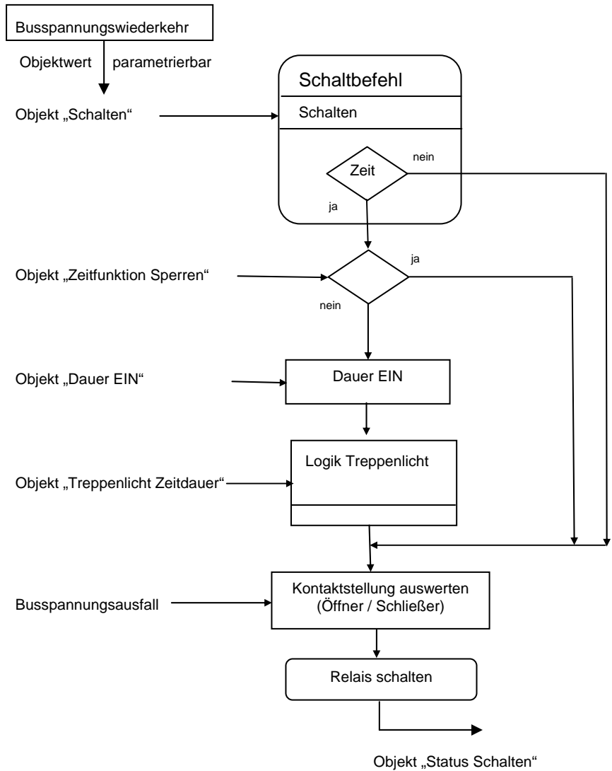
Abb. 37: Funktionsschaltbild Betriebsart Schaltaktor
