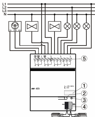
Abb. 6: Anschlussbild des Lüftungsaktors, 5stufig 6164/42
