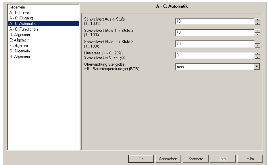
Abb. 12: Parameterfenster " A - C: Automatik"
