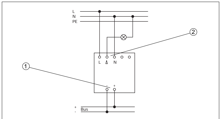
1 Busanschluss
