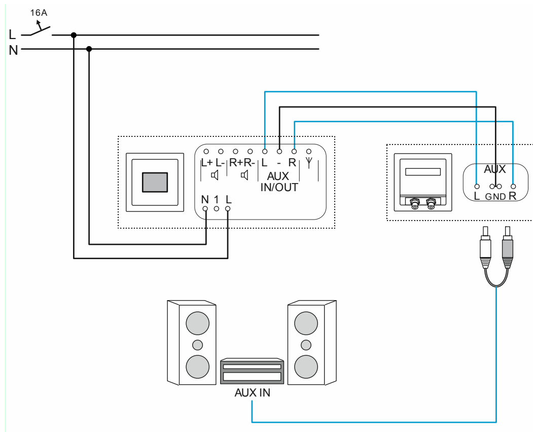
Abb. 92: Unterputz-Radio mit HiFi-Anlage: Anschluss
