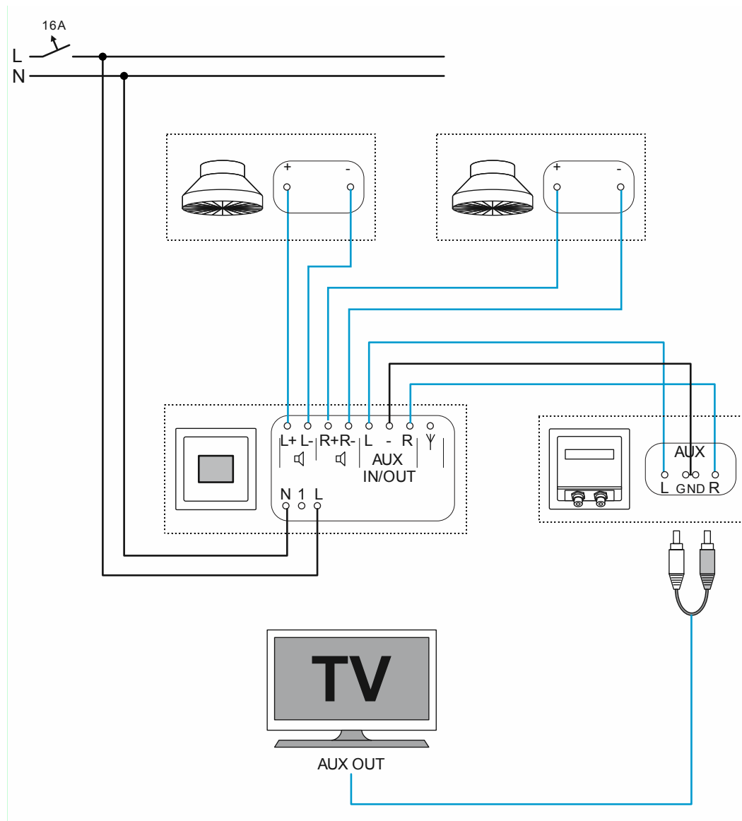
Abb. 96: Unterputz-Radio mit TV: Anschluss
