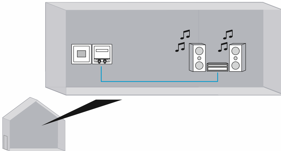
Abb. 91: Unterputz-Radio mit HiFi-Anlage: Übersicht
