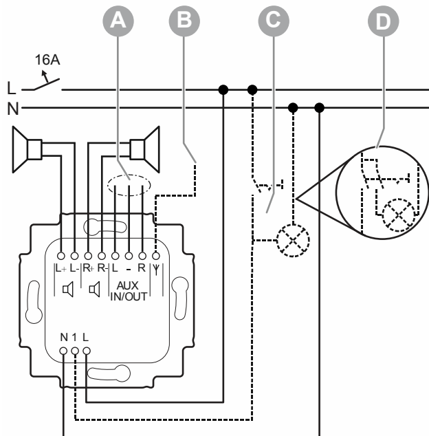
Abb. 8: Elektrischer Anschluss
