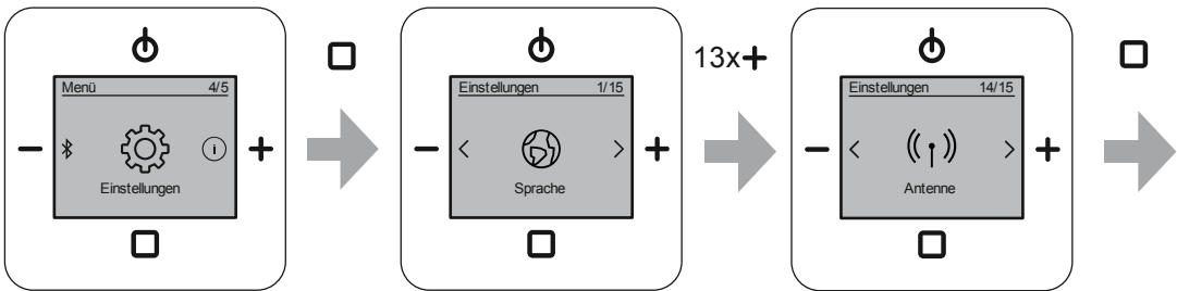
Abb. 74: Antenne
