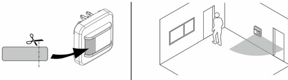
Abb. 14: Einschränkung Erfassungsbereich: Selectlinse
