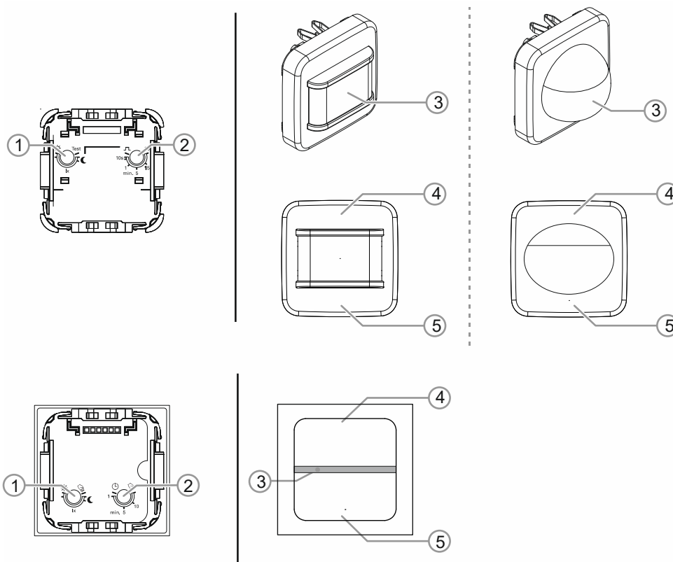
Abb. 20: Bedienelemente
