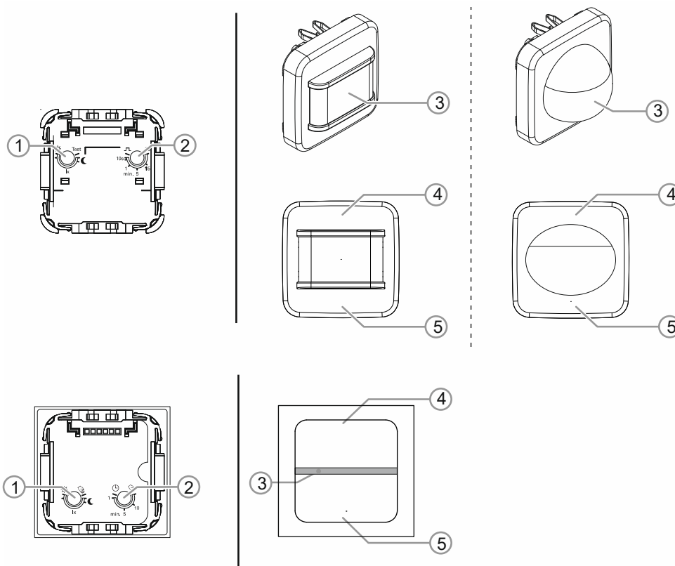
Abb. 21: Bedienelemente
