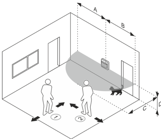
Abb. 10: Erfassungsbereiche: Prinzip Selectlinse
