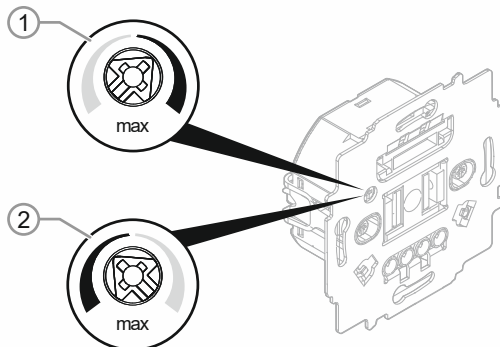
Abb. 23: Einstellung minimale Helligkeit
