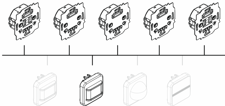
Abb. 6: 180 flex, Komfort Sensor mit Selectlinse: Funktionen in Kombination mit UP-Einsätzen
