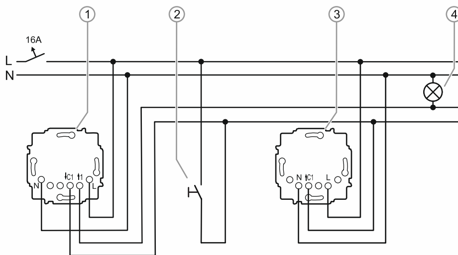
Abb. 19: Anschlussbeispiel: Hauptstelle mit Nebenstelle und Nebenstellentaster
