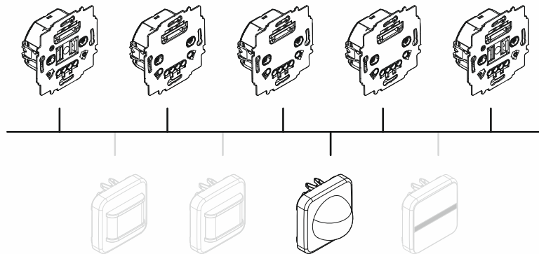
Abb. 7: 180 flex, Komfort Sensor mit Multilinse: Funktionen in Kombination mit UP-Einsätzen
