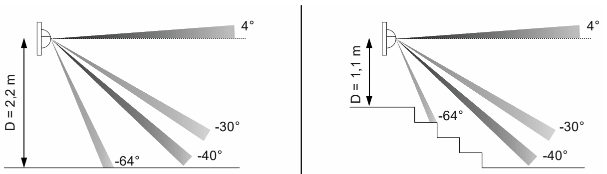
Abb. 15: Öffnungswinkel Multilinse
