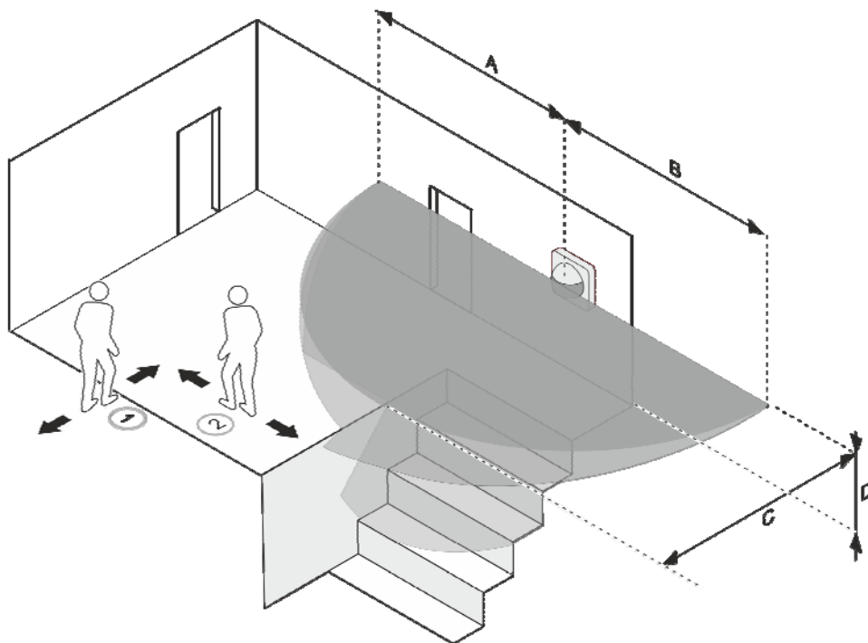
Abb. 16: Erfassungsbereiche: Prinzip Multilinse
