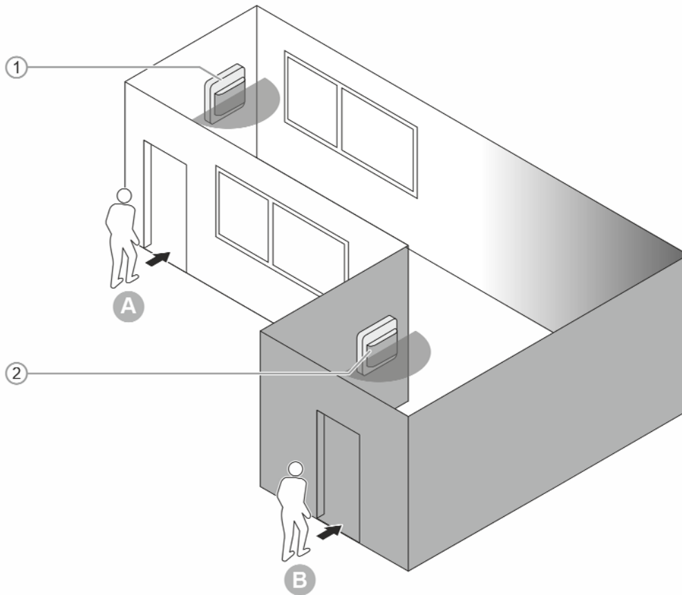
Abb. 32: Anwendungsbeispiel: Korridor mit hellen und dunklen Bereichen
