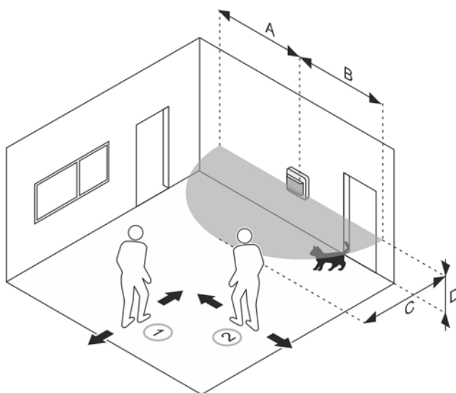
Abb. 13: Erfassungsbereiche: Prinzip Selectlinse
