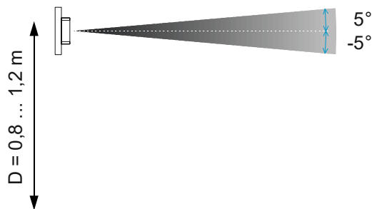
Abb. 12: Öffnungswinkel Selectlinse
