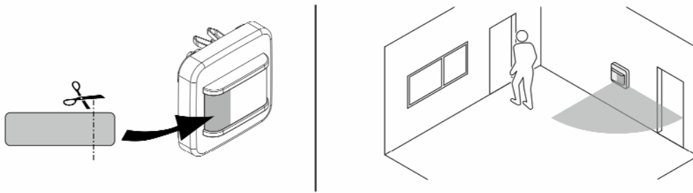
Abb. 11: Einschränkung Erfassungsbereich: Selectlinse
