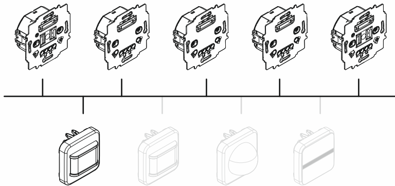
Abb. 5: 180 flex, Basic Sensor mit Selectlinse: Funktionen in Kombination mit UP-Einsätzen
