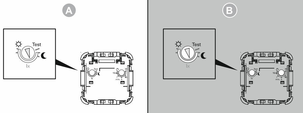
Abb. 33: Anwendungsbeispiel: Korridor mit hellen und dunklen Bereichen – Einstellen der Helligkeitsschwelle
