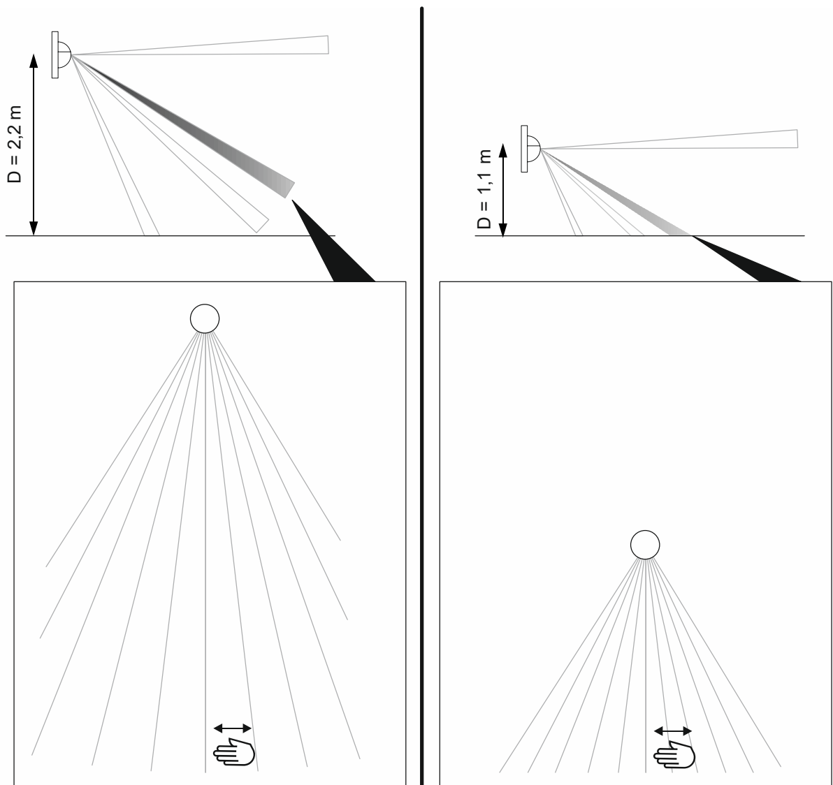
Abb. 31: Montagehöhen
