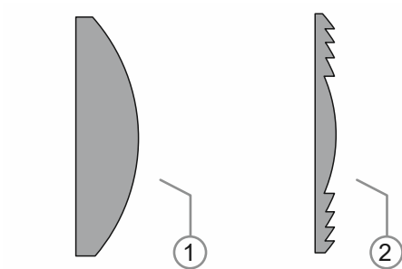
Abb. 28: Linsenarten
