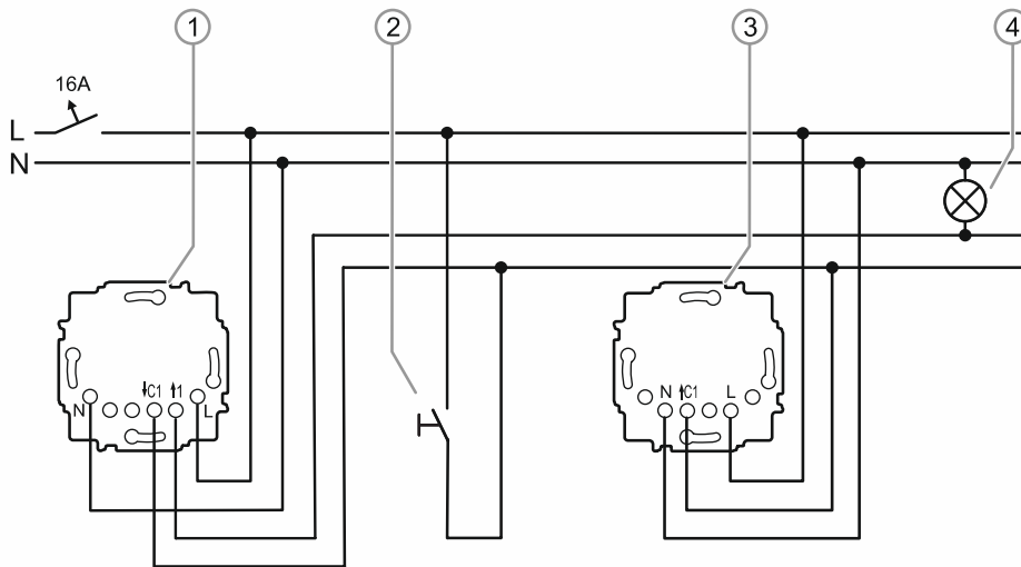
Abb. 34: Anwendungsbeispiel: Korridor mit hellen und dunklen Bereichen – Anschluss
