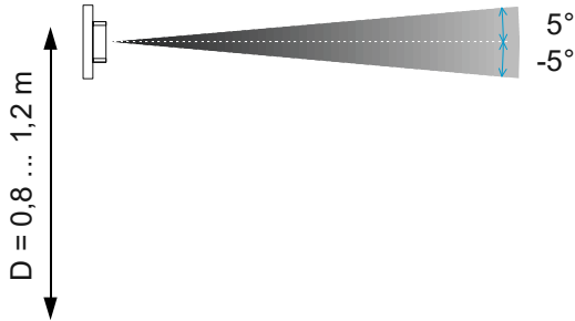
Abb. 9: Öffnungswinkel Selectlinse
