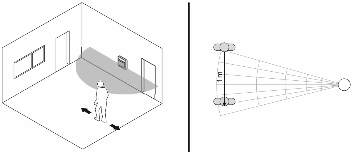
Abb. 29: Erfassung quer zum Gerät
