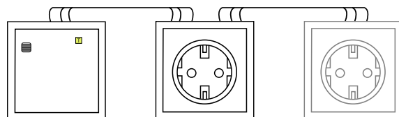
FI-Schalter mit normalen Steckdosen unter verschiedenen Abdeckungen – erlaubt
