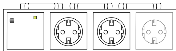
FI-Schalter mit normalen Steckdosen unter einer gemeinsamen Abdeckung – erlaubt
