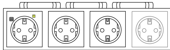
FI-Steckdose mit normalen Steckdosen unter einer gemeinsamen Abdeckung – erlaubt
