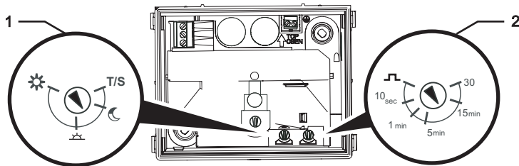
Abb. 11: Bedienelemente
