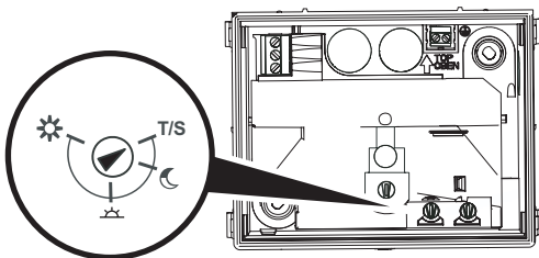
Abb. 10: Bedienelement
