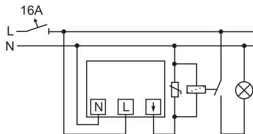
Abb. 8: Universal-Relais-Einsatz mit RC-Löschglied 6899 und Relais
