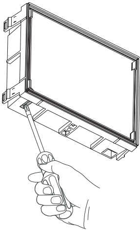
Abb. 4: Wasserablauf öffnen
