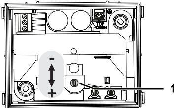
Abb. 9: Einstellung Reichweite
