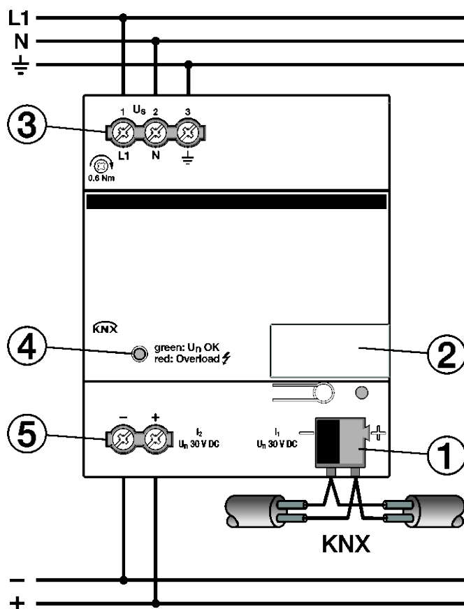
Anschlussbild
