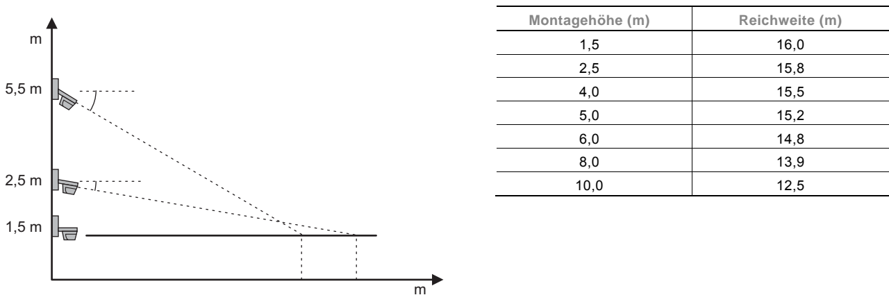
Abb. 10: Reichweitenverlust in Abhängigkeit der Montagehöhe
