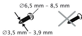
Abb. 15: Montageschrauben
