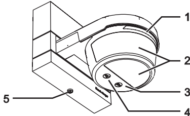
Abb. 1: Bedienelemente
