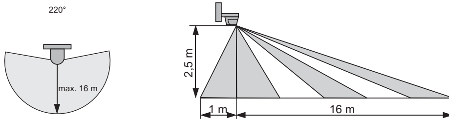
Abb. 9: Reichweite
