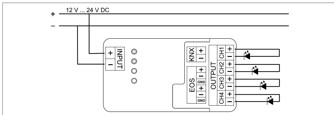
Abb. 4: Elektrische Anschlüsse
