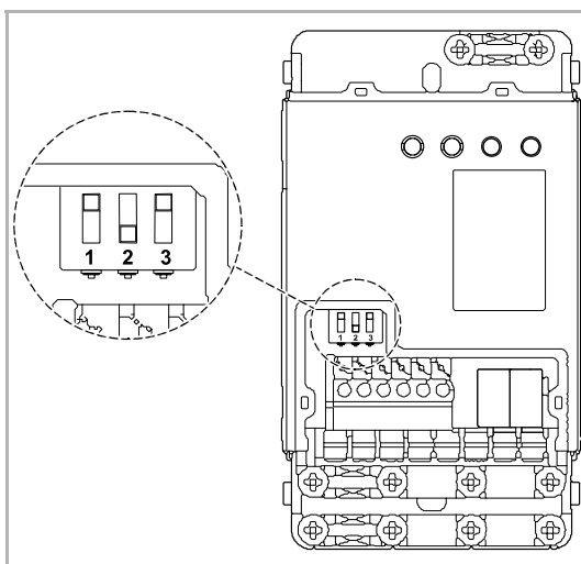
Abb. 7: DIP-Schalter
