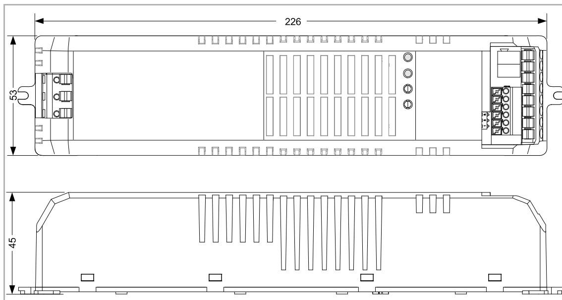
Fig. 3: Dimensioni (tutte le misure in mm)
