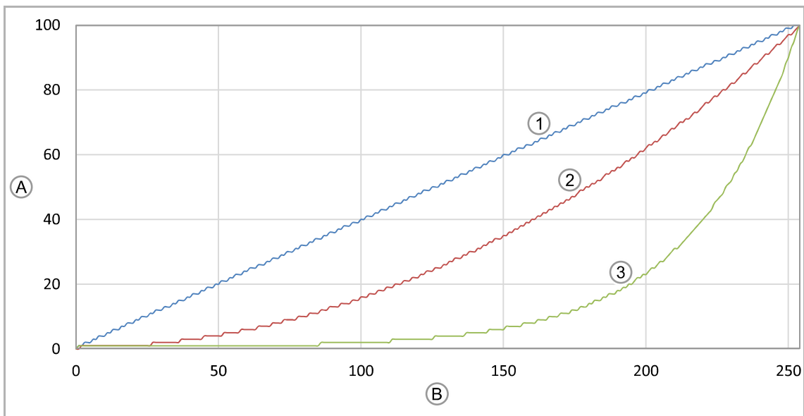
Abb. 8: Vergleich Dimm-Kurven
