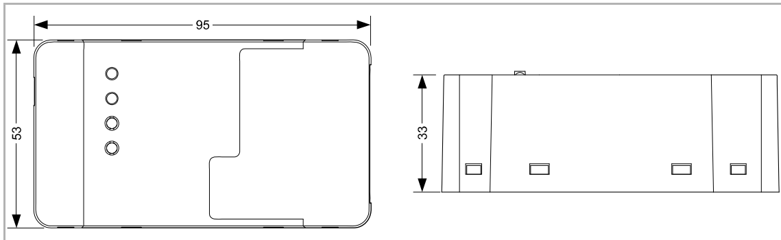
Abb. 3: Abmessungen (alle Maße in mm)
