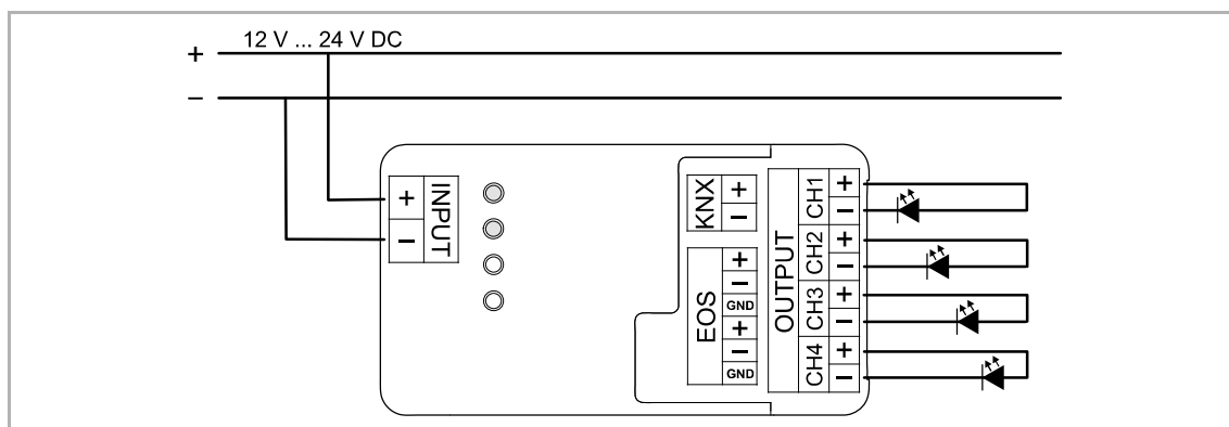
Abb. 4: Elektrische Anschlüsse
