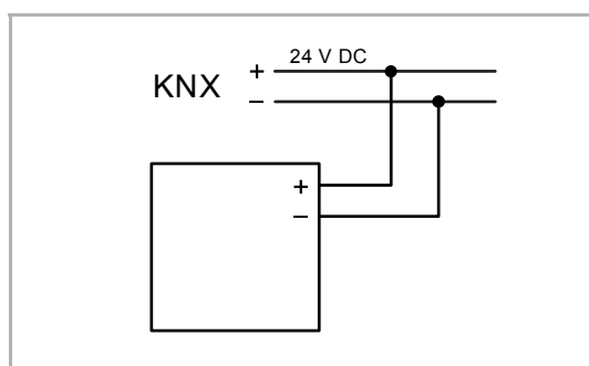
Abb. 5: Anschluss Busankoppler
