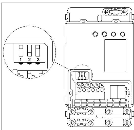
Abb. 7: DIP-Schalter
