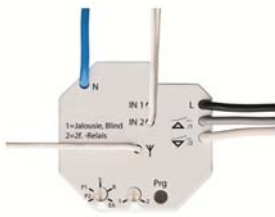
Serien-/Jalousieaktor WaveLINE Artikel-Nr. 6705-101
