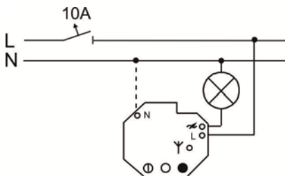
Universal-Dimmaktor WaveLINE Artikel-Nr. 6704
