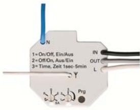
1-fach Aktor WaveLINE Artikel-Nr. 6702
