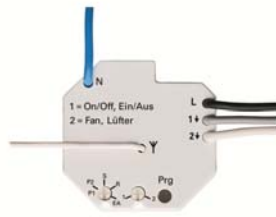
2-fach Aktor WaveLINE Artikel-Nr. 6703
