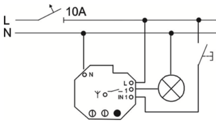
Schaltaktor WaveLINE, 1-fach, mit Nebensstelle Artikel-Nr. 6701-101
