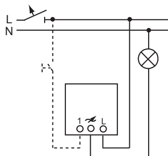
Universal-Dimmer-Einsatz Artikel-Nr. 6595 U
