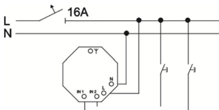
Binäreingang WaveLINE, 2-fach Artikel-Nr. 6725
