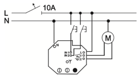
Serien-/Jalousieaktor WaveLINE Funktion als Jalousieaktor Artikel-Nr. 6705-101
