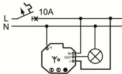
Schaltaktor WaveLINE Artikel-Nr. 6702
