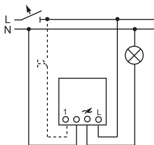
Universal-Relais-Einsatz Artikel-Nr. 6404 U
