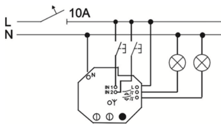
Serien-/Jalousieaktor WaveLINE Funktion als Serienschaltaktor Artikel-Nr. 6705-101
