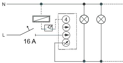
Рис. 4: Выключение выключателем деблокировки сетевого питания
